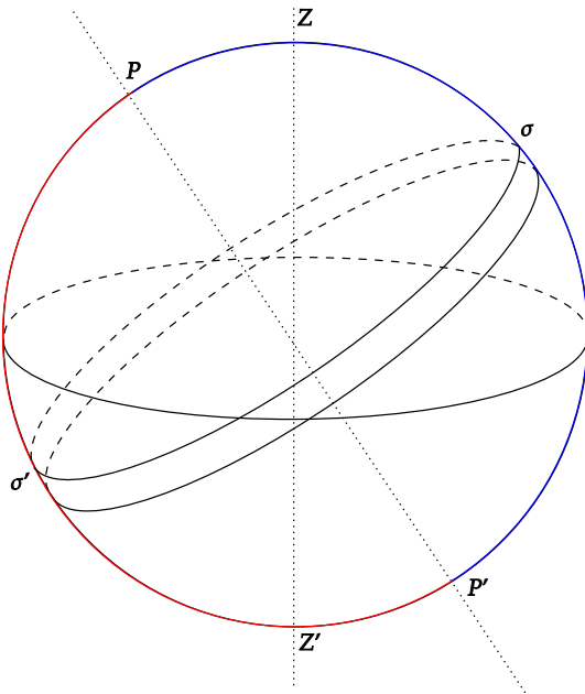
图 3.2: \sigma 是上中天, \sigma' 是下中天
